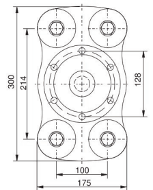
Aquadrive CVB 30.20 (kuva yllä) nivelen pituus 245mm, Ø148 esim. 270hv / 3300rpm, välitys 2:1, max 2000rpm
