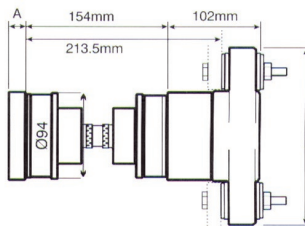
Aquadrive CVB 10.10 esim. 85hv / 3800rpm, välitys 2:1, max 4000rpm A (Adapterilaiippa) ~25mm
