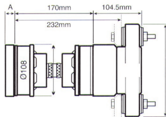
Aquadrive CVB 15.10 (kuva vasemmalla) esim. 155hv / 3800rpm, välitys 2:1, max 4000rpm A (Adapterilaiippa) ~30mm
